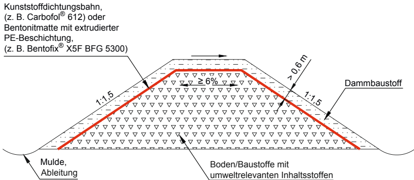
Abbildung 5: Wall für die Bauweise C mit witterungsunempfindlicher Abdichtungskomponente
