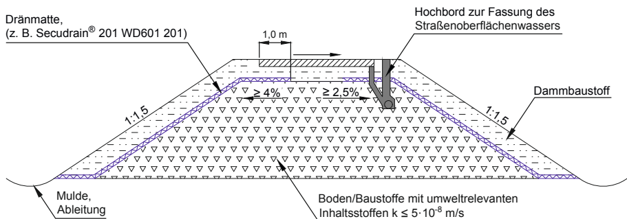
Abbildung 7: Ausführungsvorschlag für einen Damm in Bauweise E (Variante 1) mit Geokunststoffen
