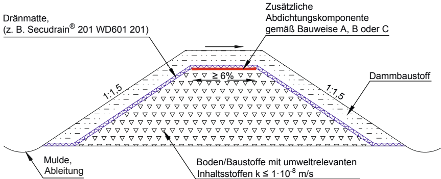
Abbildung 9: Ausführungsvorschlag für einen Wall in Bauweise E (Variante 2) mit Geokunststoffen
