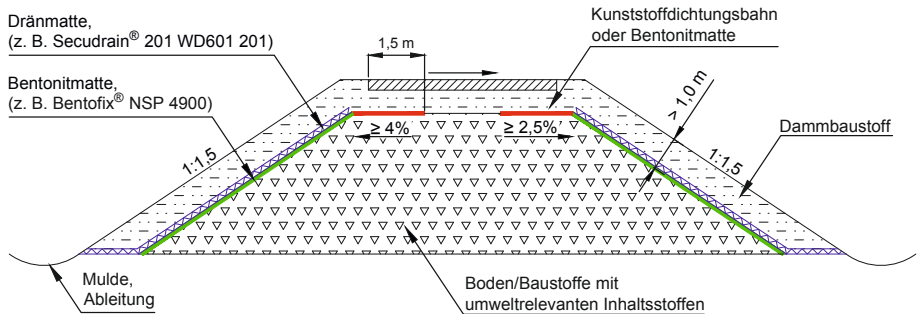
Abbildung 3: Ausführungsvorschlag für die Bauweise B mit Geokunststoffen
