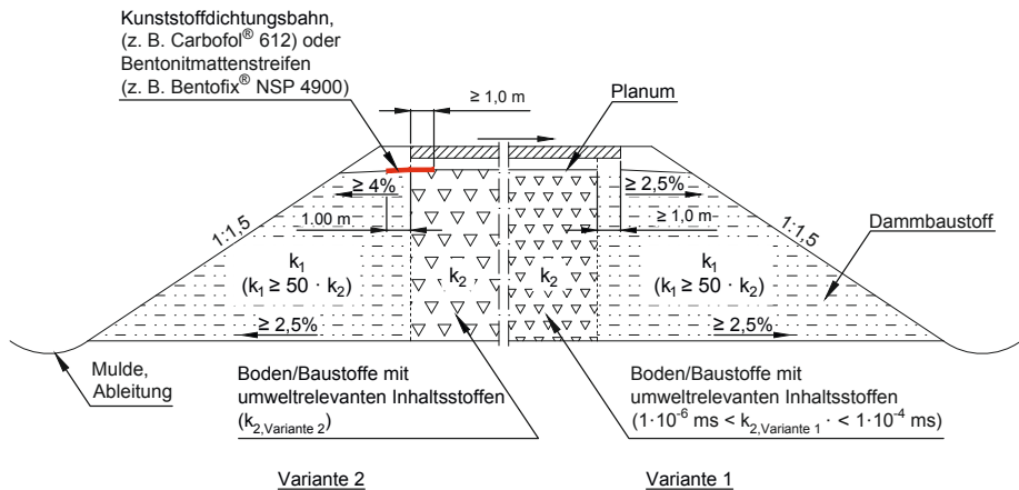
Abbildung 6: Damm mit Kern aus Boden oder Baustoff mit umweltrelevanten Inhaltsstoffen - Varianten der Bauweise D zur Vermeidung eines kapillaren Wassertransportes im Kern, mit eingrücktem Kern (rechts), bzw. Variante 2 mit Abdichtungsstreifen (links)
