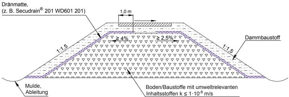
Abbildung 8: Ausführungsvorschlag für einen Damm in Bauweise E (Variante 2) mit Geokunststoffen
