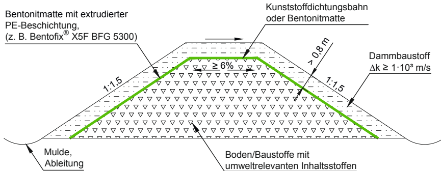
Abbildung 2: Ausführungsvorschlag für einen Wall in Bauweise A mit Geokunststoffen, Damm mit witterungsempfindlichen Abdichtungskomponenten ohne Sickerschicht
