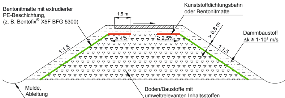
Abbildung 1: Ausführungsvorschlag für einen Damm in Bauweise A mit Geokunststoffen, Damm mit witterungsempfindlichen Abdichtungskomponenten ohne Sickerschicht
