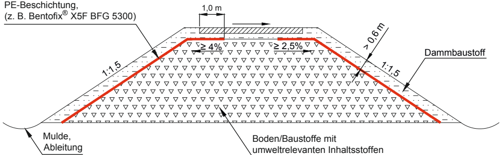
Abbildung 4: Ausführungsvorschlag für einen Damm für die Bauweise C mit Geokunststoffen
